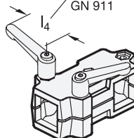
Regulowana dźwignia ręczna GN 911
